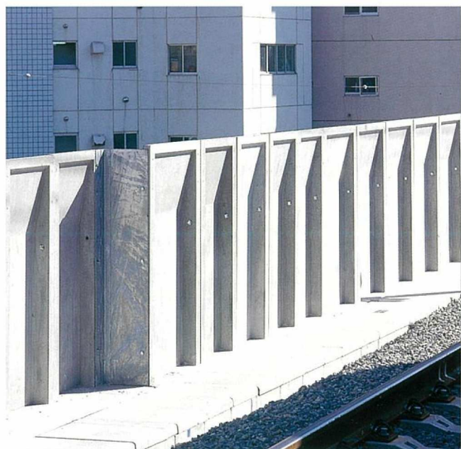
NJ軽量高欄取付状況 (同上 線路側から)
