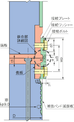
PHC杭+SC杭の例
