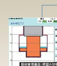
計測した油流量を拡大径に変換して表示し、あらかじめ設定しておいた計画掘削形状と比較してビジュアル的に施工管理を行います。
