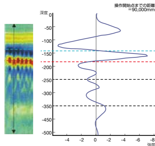
電磁波調査 当社独自の解析方法でコンクリートの内部変状が捉えられます。
